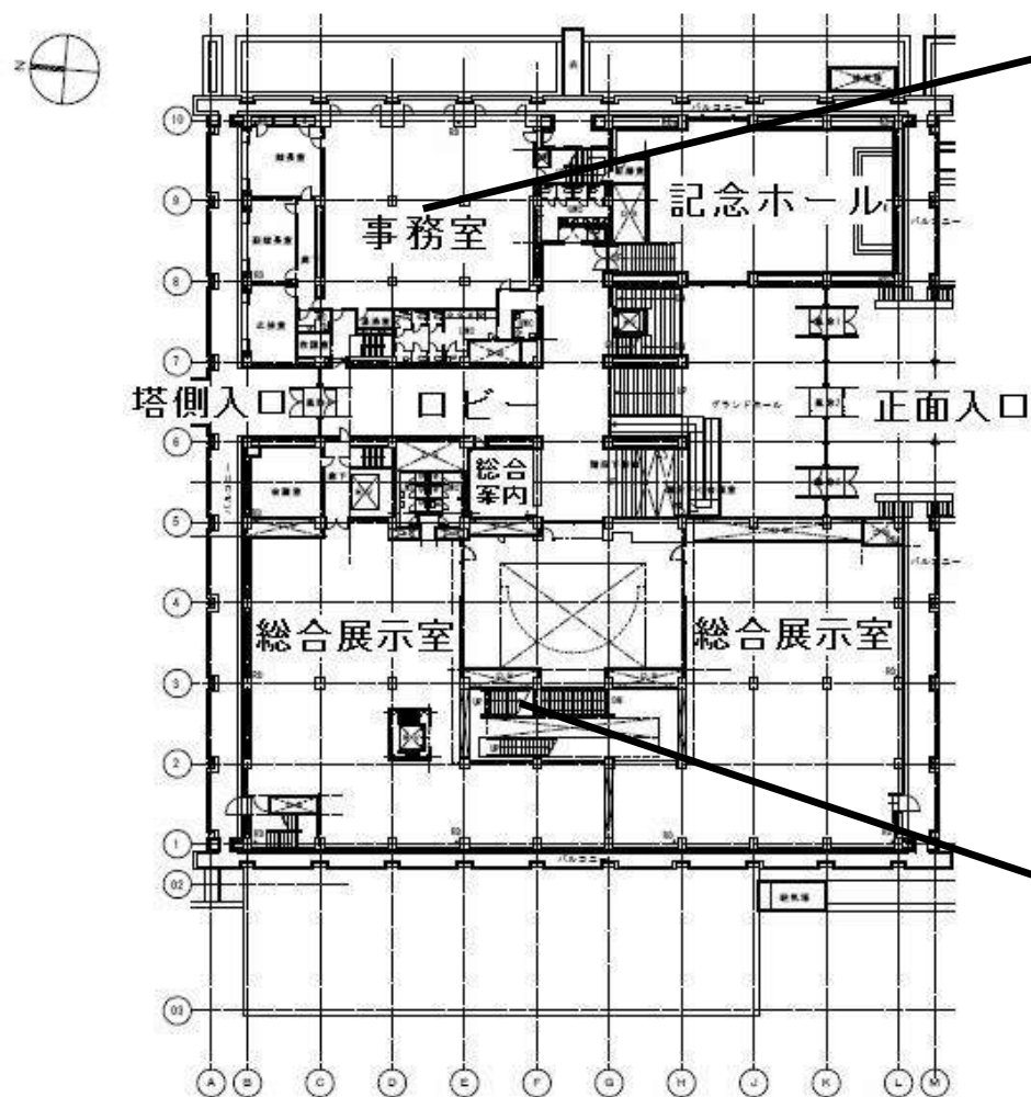
1階 (1F) 平面図
