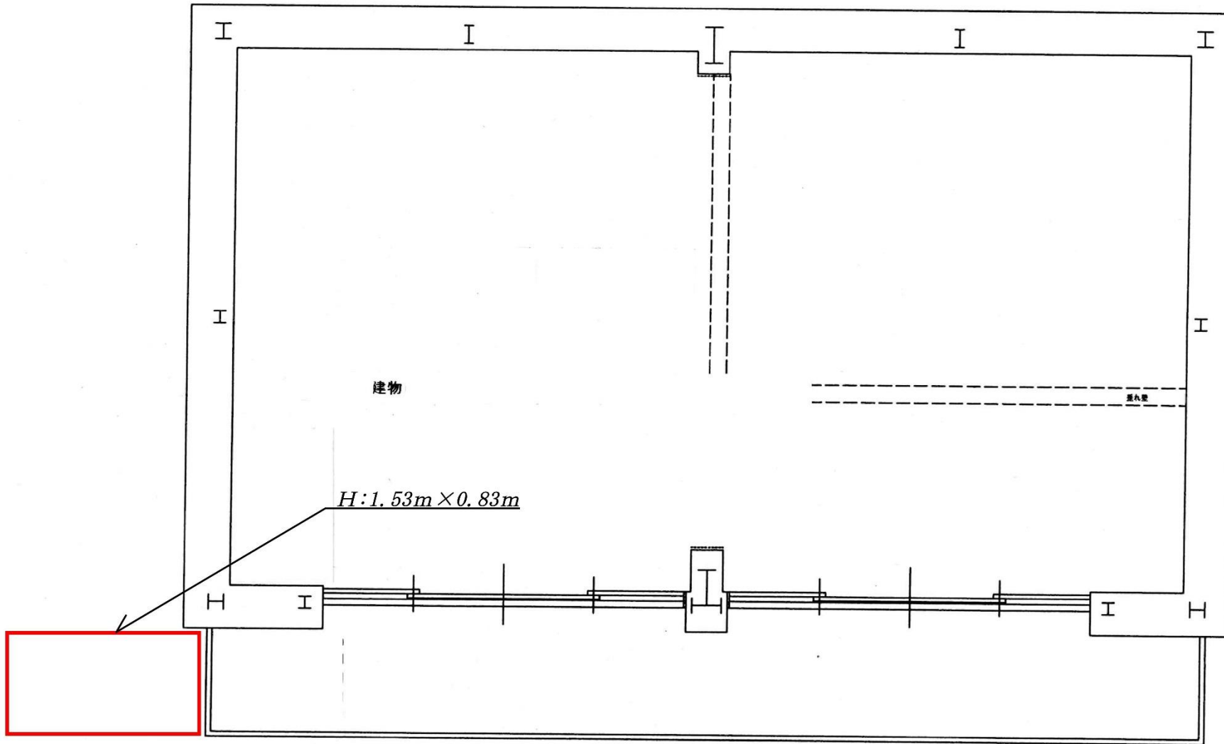
開拓の村軽飲食食堂周辺平面図
